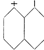
Schöllkopfsche Säure. D.R.P. 40 571. Erdmann. Annal. 247. 348.
